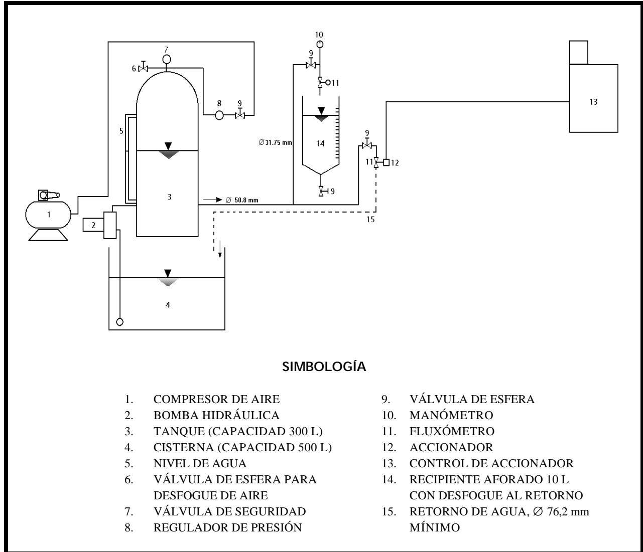
FIGURA 2. DISPOSITIVO DE PRUEBA PARA PRESIÓN HIDROSTÁTICA, VOLUMEN, TIEMPO DE DESCARGA Y DURABILIDAD
