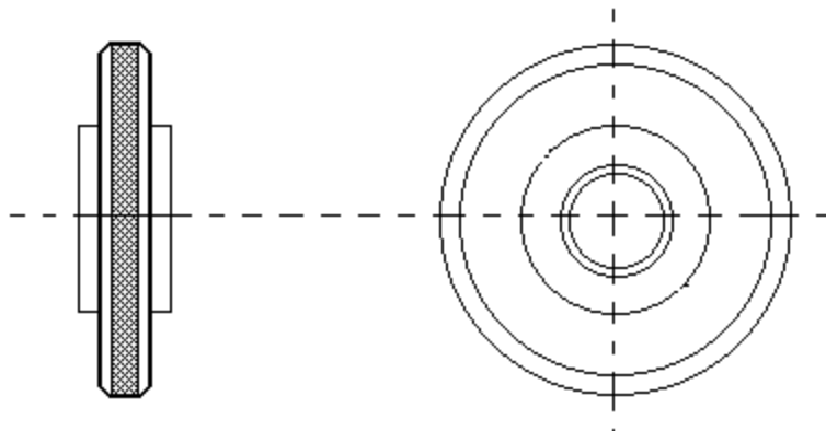
CALIBRADOR HEMBRA (ANILLO)
