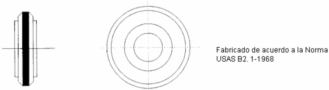
Figura 4. Calibrador hembra
